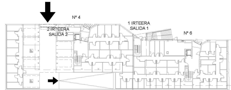
GARAJEA / GARAJE. SOTOA -1 / SÓTANO -1
