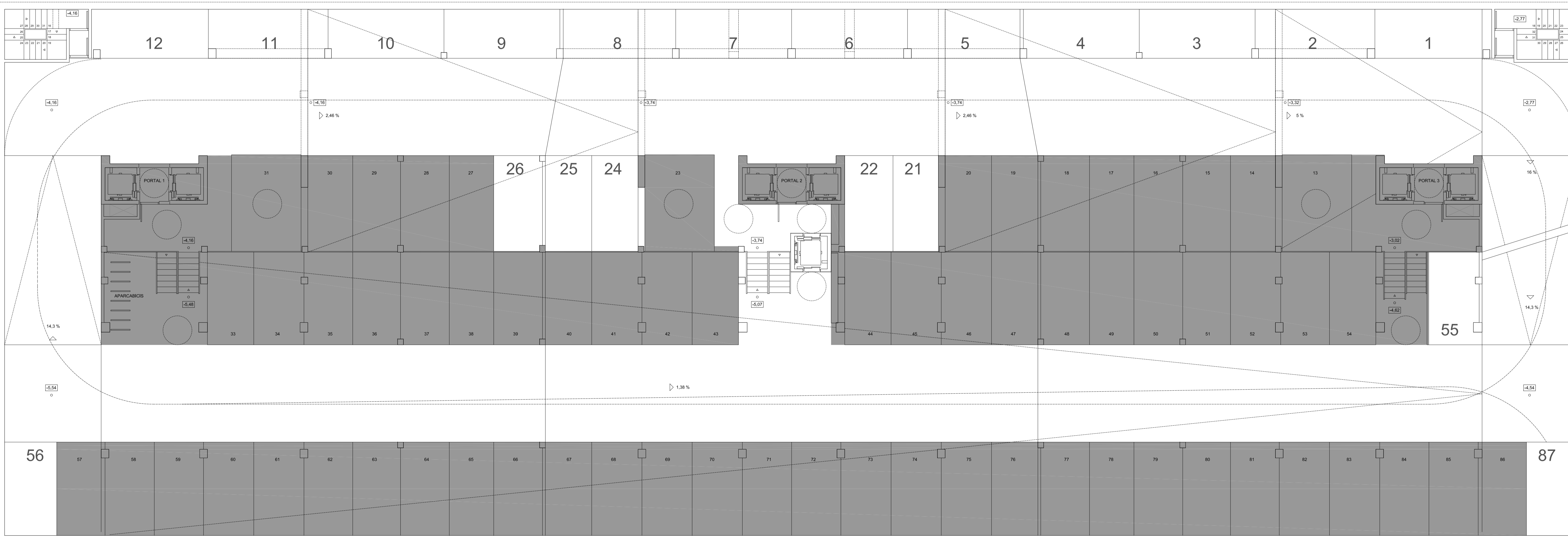
PLANTA SOTANO -1
