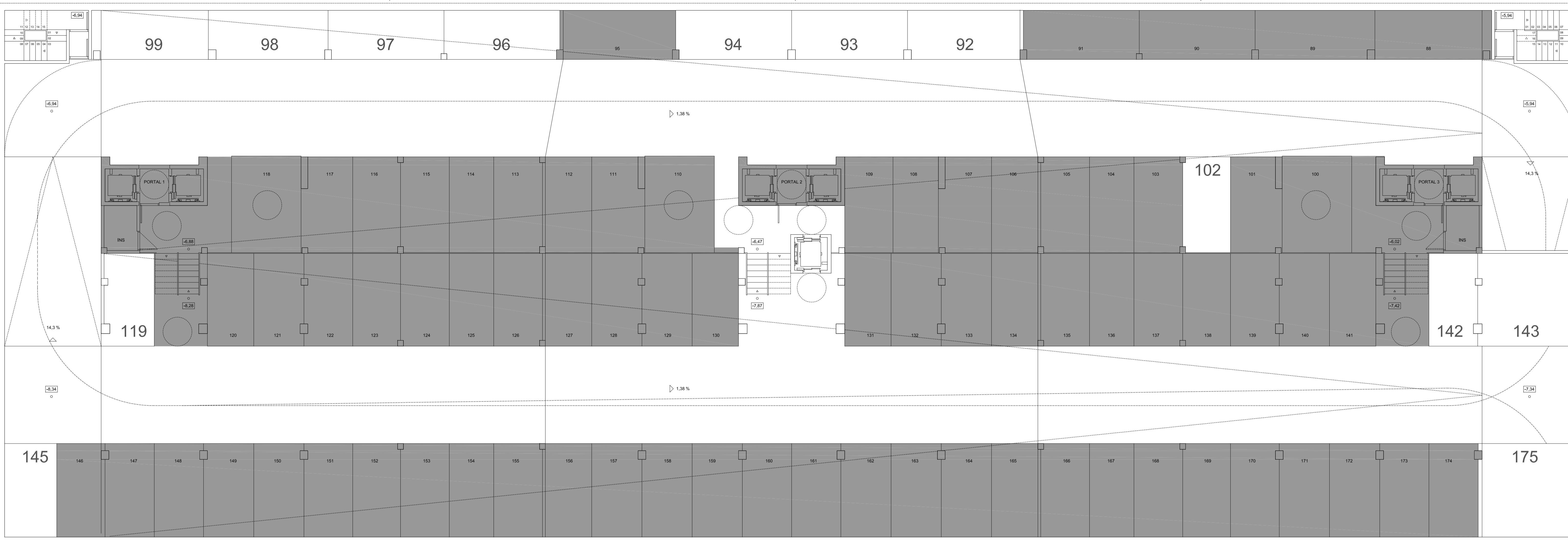
PLANTA SOTANO -2
