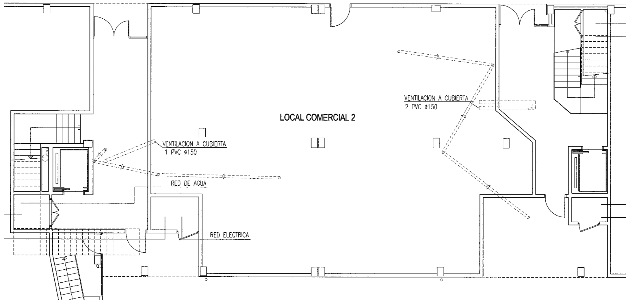
PLANTA BAJA LOCAL COMERCIAL-MERKATARITZA LOKALA E. 1/100
